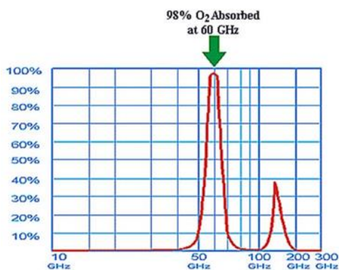
Atmosférická absorpce 60GHz vln v suché atmosféře na 1 kilometr
