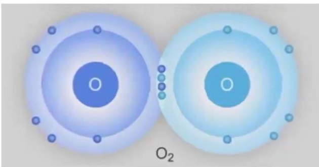
Molekula kyslíku
